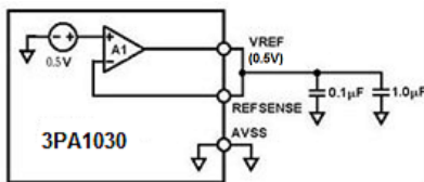
d. 0.5 V Reference
