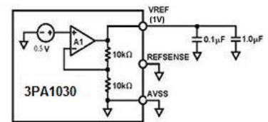
e. 1 V Reference
